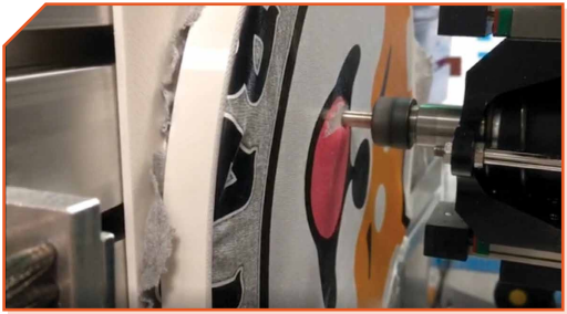
Robotic Material Preparation Device Using Tactile and Visual Guidance 以觸覺和視覺導引的材料準備機械人
