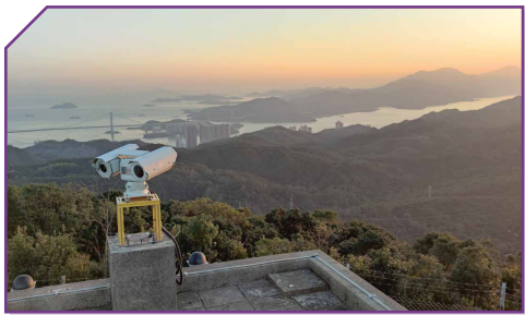
Automated Hill Fire Surveillance System 自動山火監控系統
